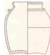
图四 陶罐(1:5)
