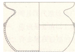
图二 铜釜(1:5)
